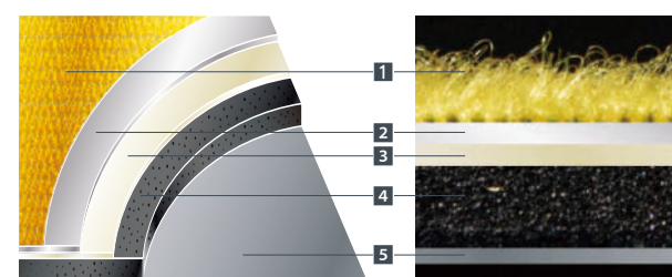
AGTitan210 ® 五層構造
